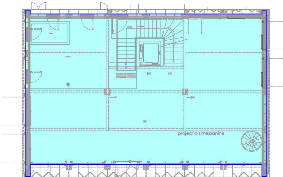
RDC Bâtiment B
